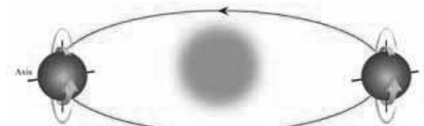
चित्र 17.24 : अपने कक्षीय पथ पर यूरेनस।
