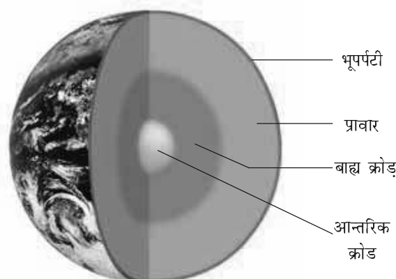
चित्र 15.9: पृथ्वी की संरचना।
