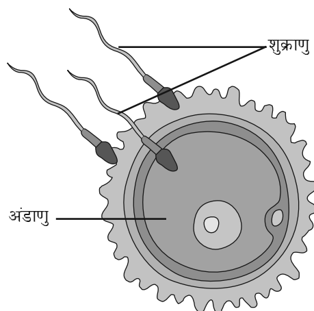
चित्र 9.5 : निषेचन।
