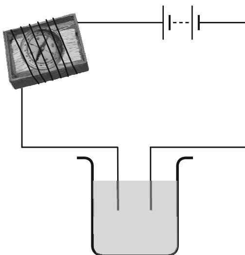
चित्र 14.9
