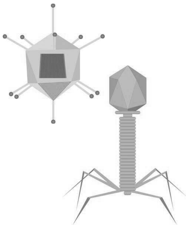
चित्र 2.5 : विषाणु।
