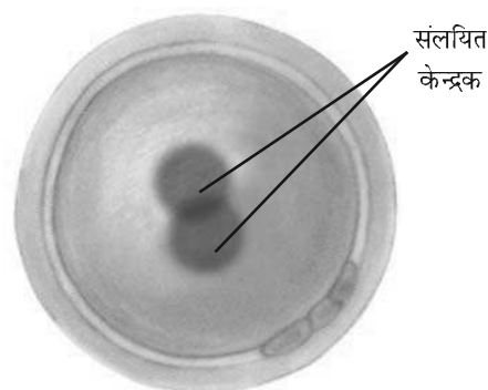
चित्र 9.6 : युग्मनज।
