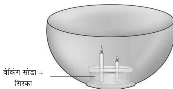
चित्र 6.15
