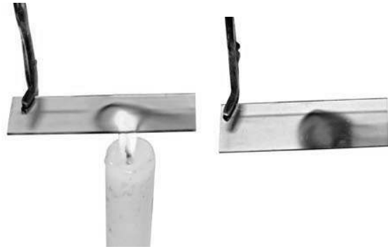
चित्र 6.11
