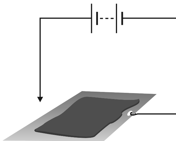
चित्र 14.11
