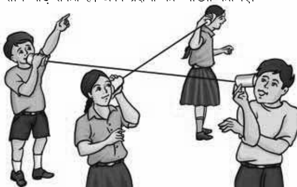
चित्र 13.20
