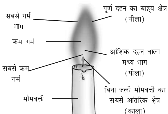
चित्र 6.13 : मोमबत्ती की ज्वाला के विभिन्न क्षेत्र।
